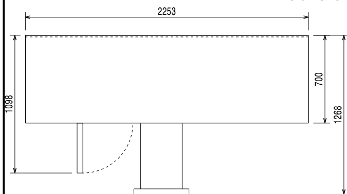
Felülnézet
